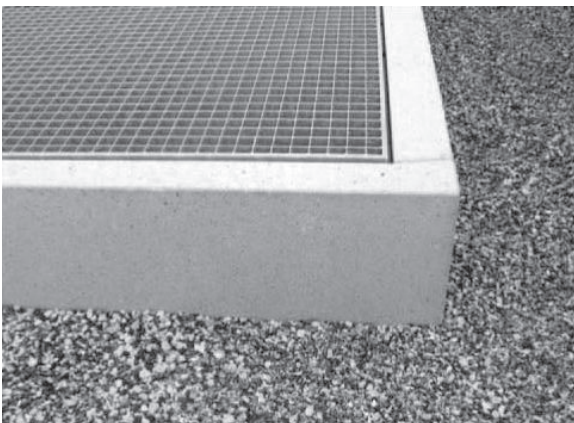
Abb. 10 Überhöhter Schachtrand
